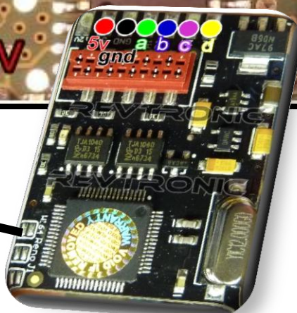
Puente para W164
