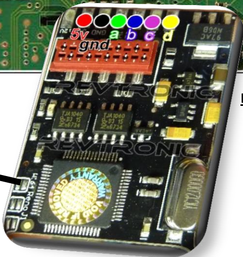
Puente para W164
