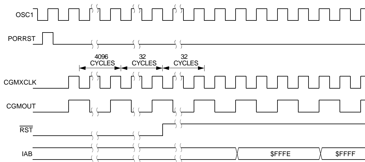
Figure 8-6. POR Recovery
